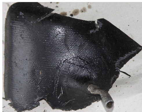
29 – Górny fragment płaszcza zbiornika paliwowego z wyprowadzeniem przewodu odpowietrzenia.
