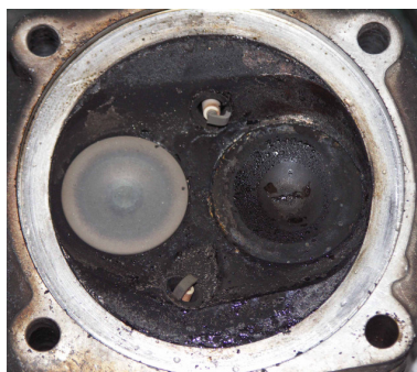
37, 38, 39 – Wnętrza zdemontowanych głowic cylindrów, widoczny stan zaworów.
