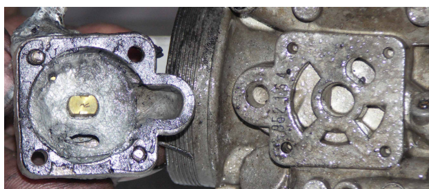
57 i 58 – Jeden z gaźników po demontażu – po prawej zespół iglicy i dysza.
