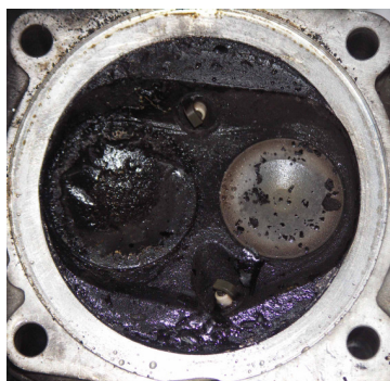
37, 38, 39 – Wnętrza zdemontowanych głowic cylindrów, widoczny stan zaworów.
