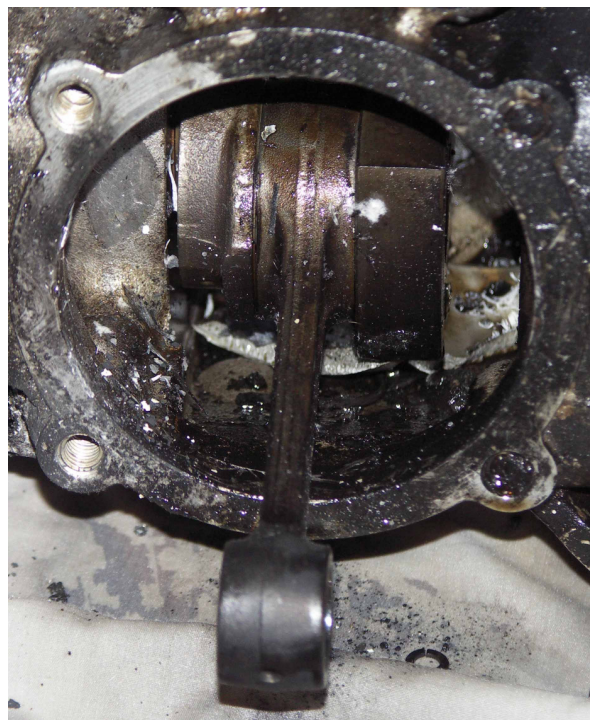
44 – Jeden z korbowodów po zdjęciu tłoka.
