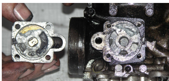
59 i 60 – Gaźniki – zdjęte sterowanie poprawką wysokości.
