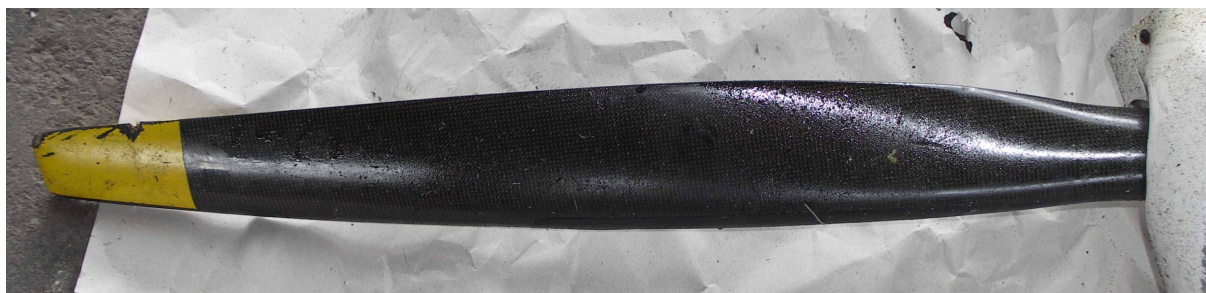
35 i 36 – Łopaty śmigła – u góry pozostająca w piaście, u dołu – oderwana. Trzecia łopata uległa złamaniu tuż przy piaście w chwili zderzenia z ziemią i dostała się pod spód silnika, po czym spłonęła.
